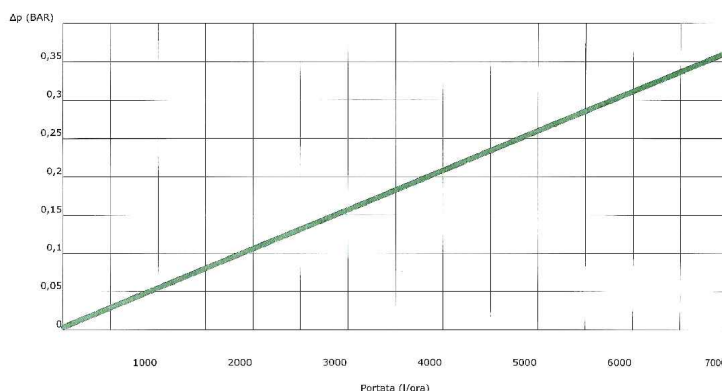
DIAGRAMMA DI PORTATA VS CADUTA DI PRESSIONE
